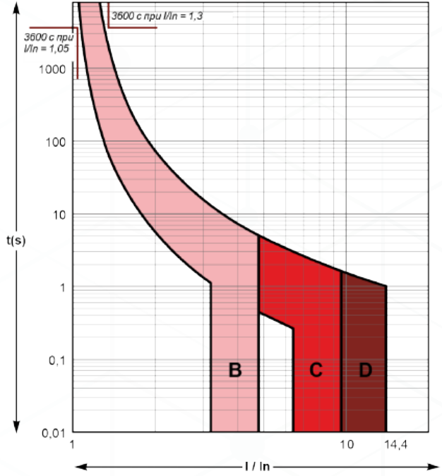
Кривые В, С, D от 6 до 125 А
