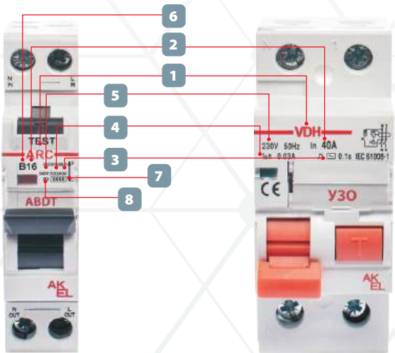
BA47-RCBO (АВДТ) BA47-RCCB (УЗО)
